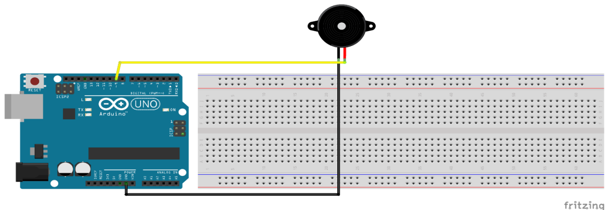
Figura 33 – Montagem do circuito elétrico
