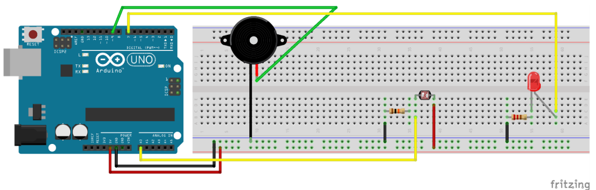
Figura 35 – Montagem do circuito Buzzer LDR + LED
