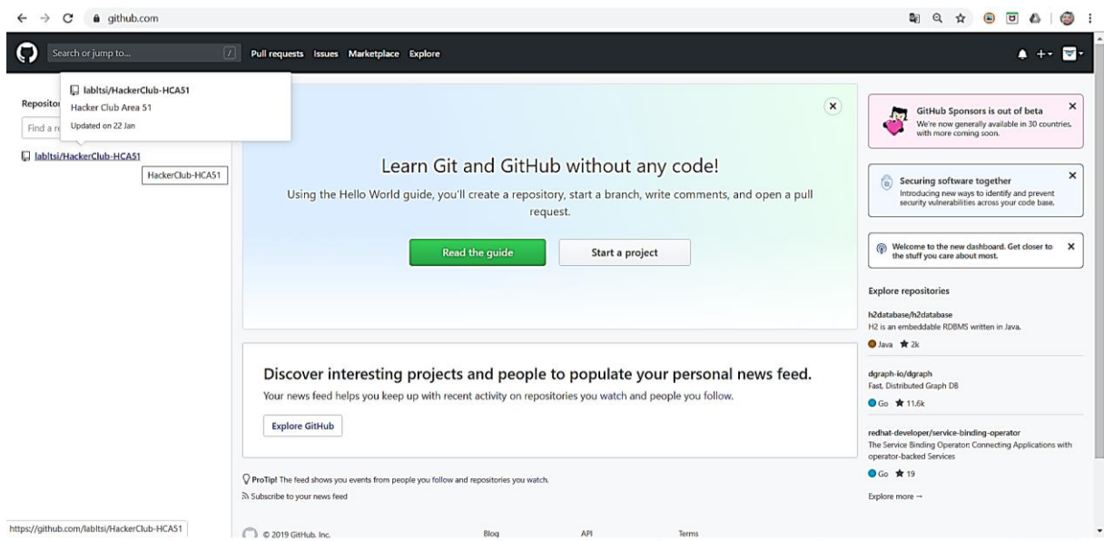
Figura 53 – Plataforma Github
