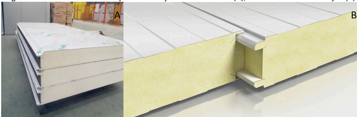
Figura 115 – Placas de isolantes para construção de Câmara Fria (A); Juntas de encaixe e fixação (B)
