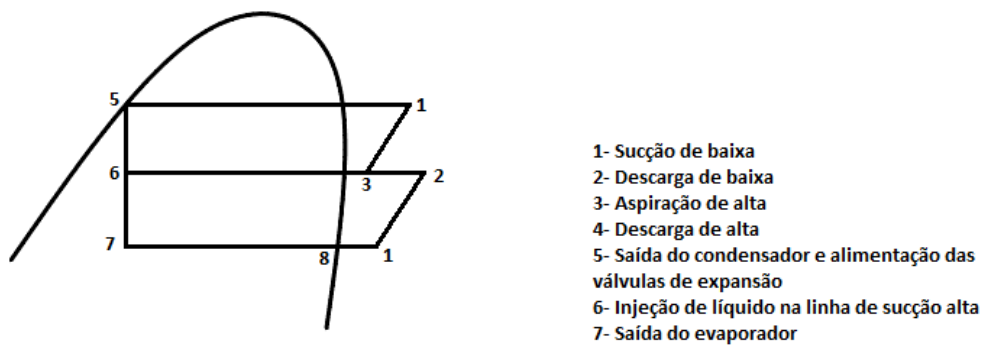
Figura 38 – Representação no diagrama pressão-entalpia e esquema de um sistema de duplo estágio com injeção de líquido na linha de aspiração
