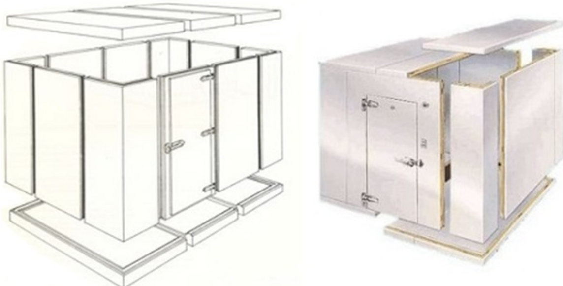
Figura 40 – Estrutura e montagem de câmara fria modular utilizando painéis pré-fabricados
