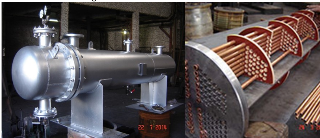
Figura 58 – Trocador de calor casco e tubo
