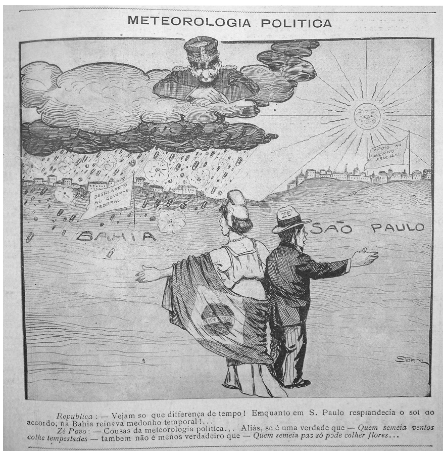
FIGURA 13. Metereologia política
