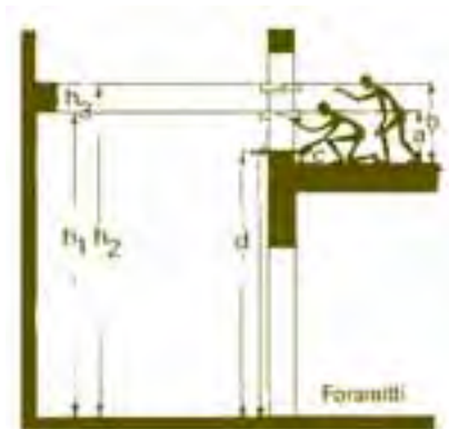
Fig. 2.16 – Transposição de pontos inacessíveis para locais acessíveis.
