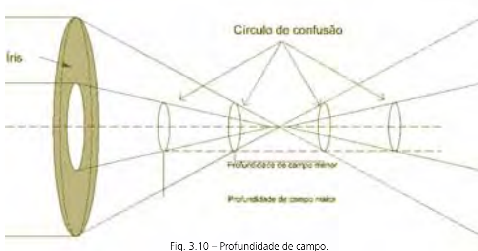
Fig. 3.10 – Profundidade de campo.
