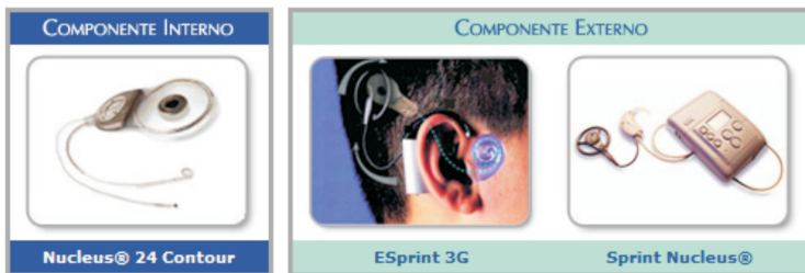
Figura 1 – componentes internos e externos de diferentes modelos de implante coclear. http://www.implantecoclear.com.br/index.php?pagina=modelos (acesso em: jun. 2010). Componentes internos: receptor estimulador com filamento de eletrodos (painel à esquerda). Componentes externos: microfone retro auricular, processador da fala, antena transmissora (painel à direita).
