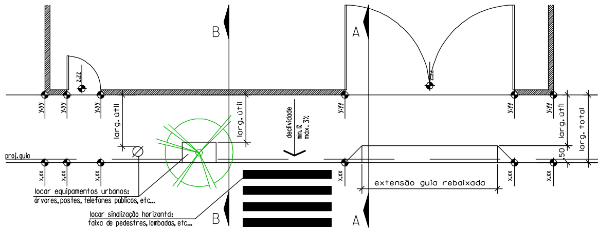
DETALHE CALÇADA - PLANTA
